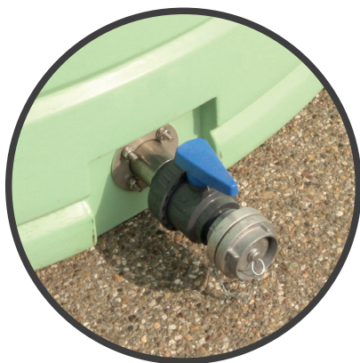
Vanne 2" (en option réf.01990900027)
