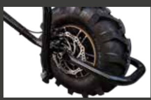
Frein à disque mécanique
