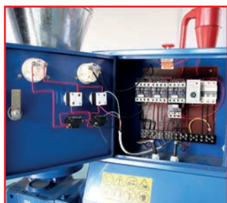
Intérieur du compartiment électrique
