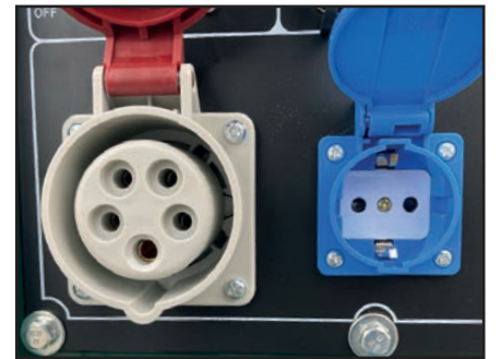
Prises 380 et 220 V
